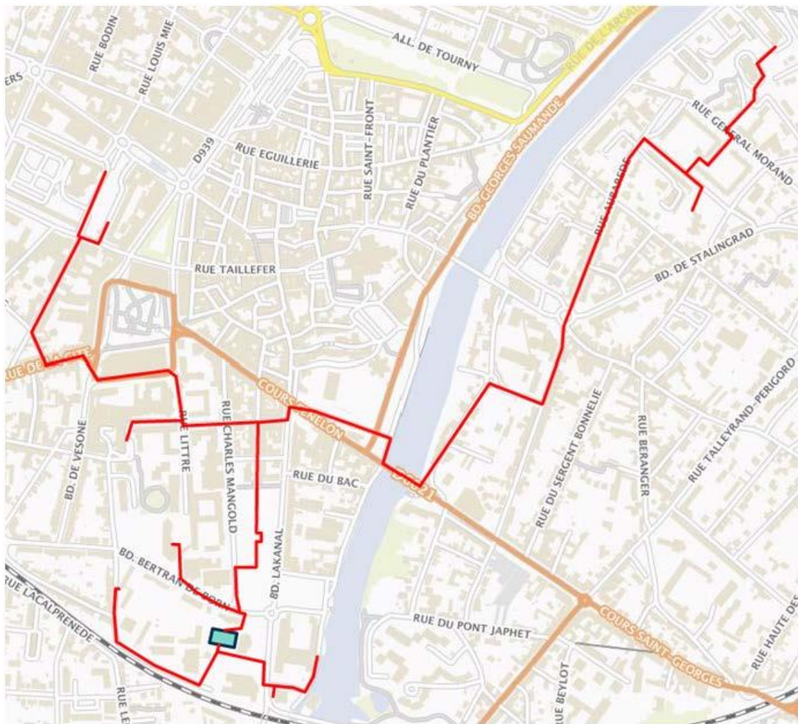
Figure 7. Tracé du réseau de chaleur des deux rives
