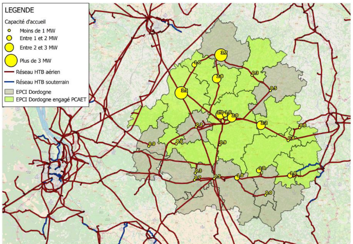
Figure 4. Capacité réservée par poste de transformation HTB/HTA au titre du S3REnR (source : RTE)
