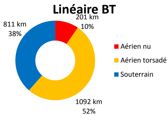
Figure 2 : CA Le Grand Périgueux - répartition du linéaire BT (source Enedis)
