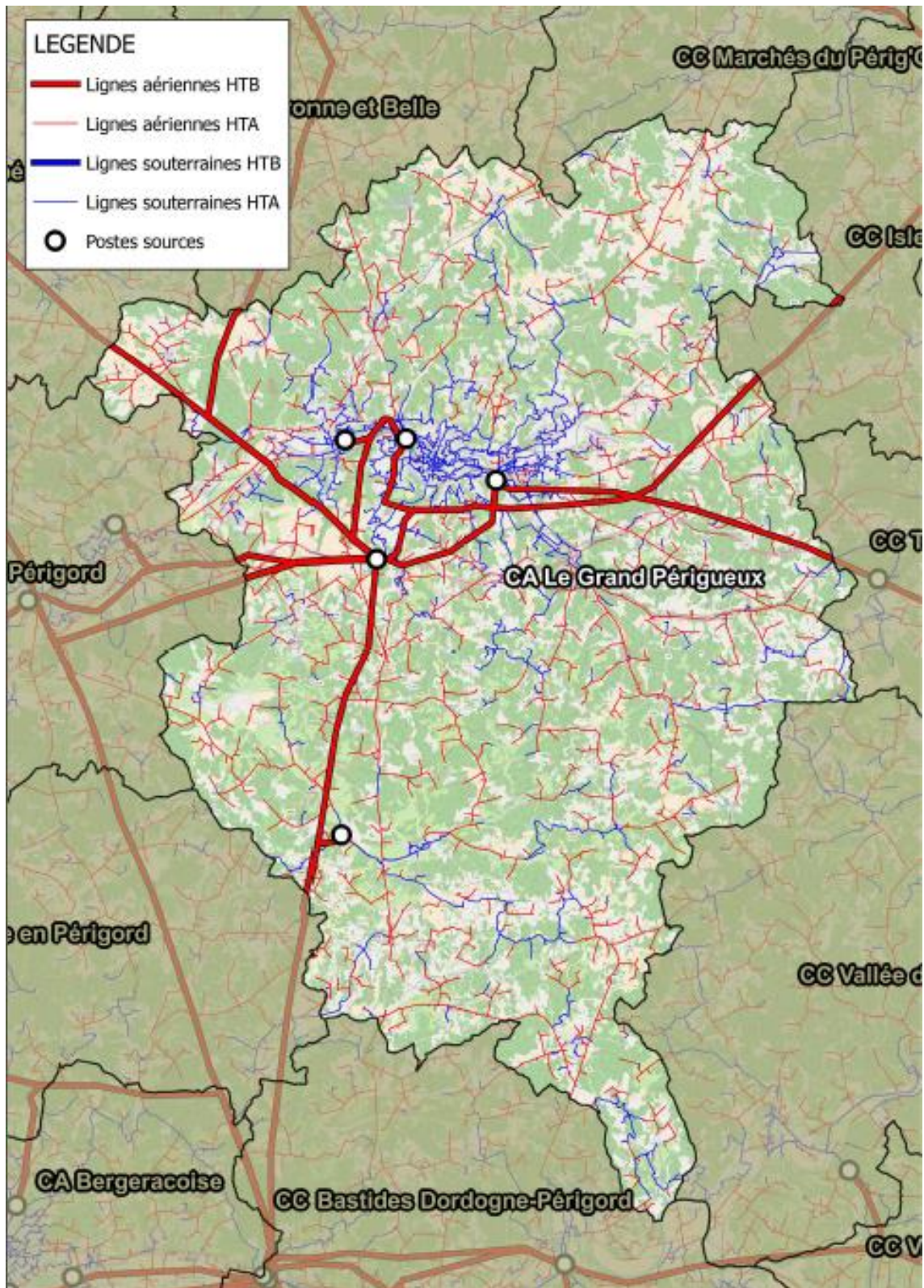
Figure 3. Cartographie des réseaux HTB et HTA sur la CA Grand Périgueux (source : RTE et Enedis)
